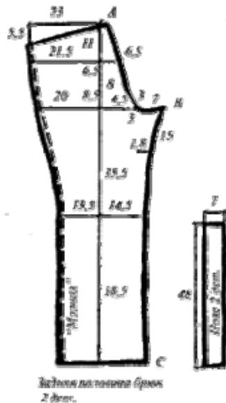
рис1. выкройка брюк 50-го размера
