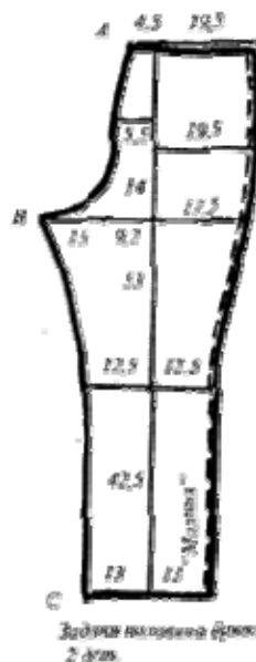
рис2. выкройка брюк 46-го размера
