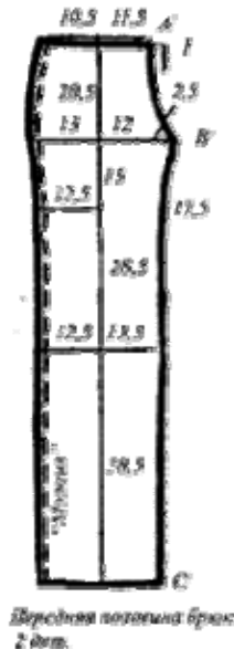
рис1. выкройка брюк 50-го размера
