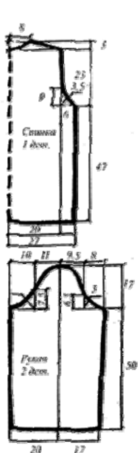
рис.1. выкройка анорака 46-го размера (без припусков на швы)
